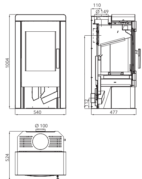
perl-schwarz, Stein Whiterock, mit Holzfach perle noir, pierre Whiterock, avec bûcher ouvert
