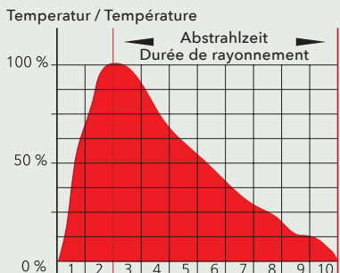
Abstrahlzeit nach dreimaligem Füllen von je 2 kg Holz Temps de rayonnement après trois charges de 2 kg de bois resp.
