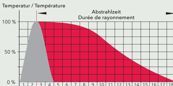
• Herkömmliche Kaminöfen / Poêles à bois conventionnels • HAAS+SOHN Wärmespeicher-Block / Bloc d'accumulation de chaleur HAAS+SOHN
